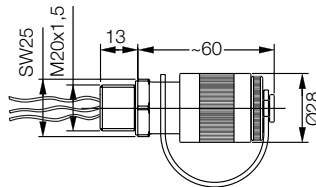
Inlet metal version: V < 2000 cm³
