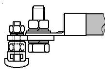
Bild 2 Sammelschienensystem - Anschluss horizontal
