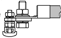
Fig. 2 Système de jeu de barres - raccordement horizontal
