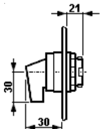
Schaltvorsatz Ex 41
