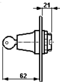
Face avant d'interrupteur à clé
