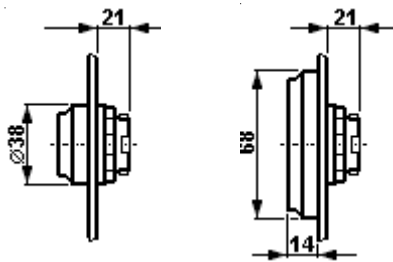
Face avant de - bouton-poussoir double bouton-poussoir
