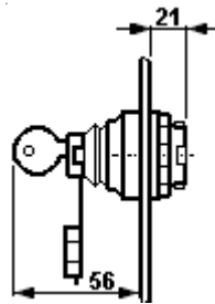
Face avant de bouton-poussoir à clé
