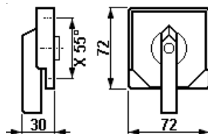
Schaltvorsatz Ex 28 / Ex 29
