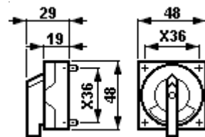
Schaltvorsatz Ex 23
