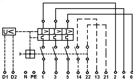
Anschlussbild - Motorschutzschalter
