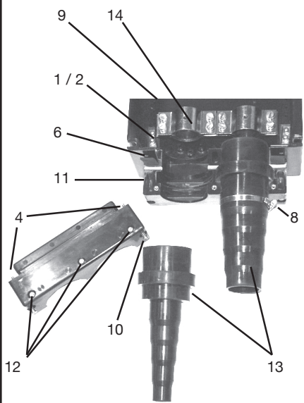
Bild 9 Montage Doppelkabelverschluss
