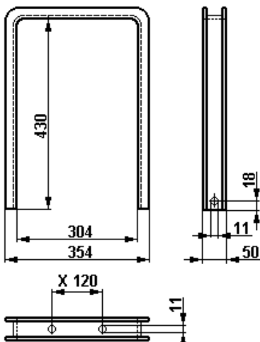
Aufhängebügel L 430
