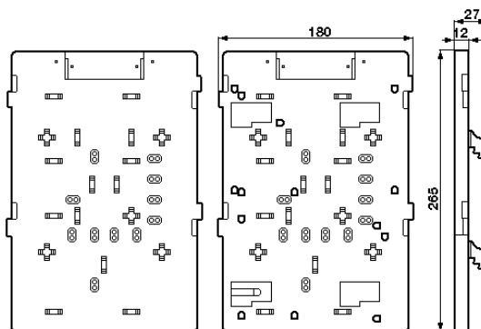
Rasthaken für Grösse 3, Lock-in hooks for size 3, Crochets à crans pour Taille 3
