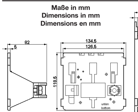
Grösse 1, Size 1, Taille 1
