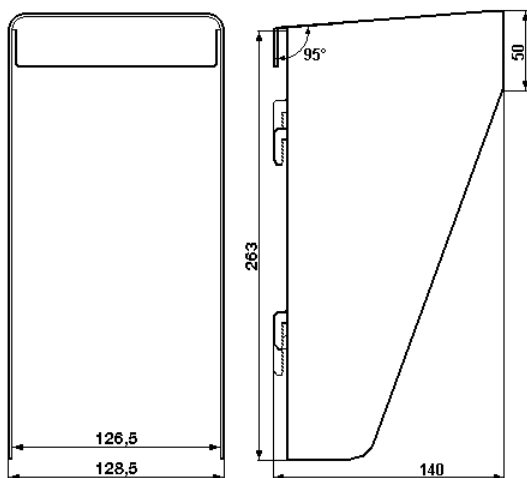
Größe 4, Size 4,• Taille 4
