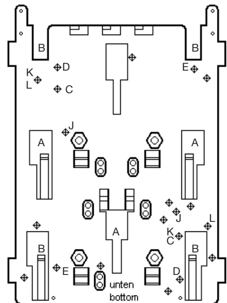
Gerätehalter für Wand- und Gitterrinnen- befestigung Apparatus holder for wall and trellis mounting Porte-appareils pour fixation au mur et au conduit de grille
