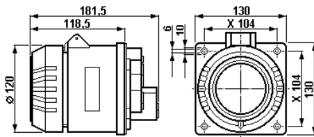
Prise encastrable
