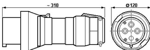
Fiche, 4- pôles
