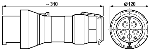
Fiche, 5- pôles
