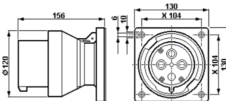
Connecteur, 4- pôles
