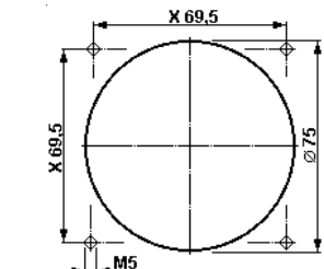
Gabarit de perçage pour connecteur
