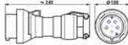
Fiche à 5 pôles
