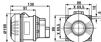
Prolongateur à 5 pôles
