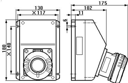
Prise murale sans interrupteur à 3- et 4 pôles
