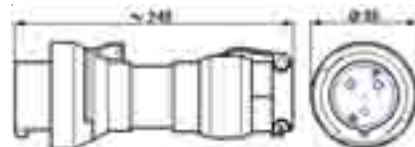
Stecker 3-polig
