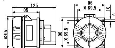
Flanschsteckdose 3- und 4-polig
