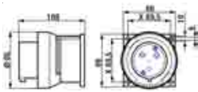
Gerätestecker 3-polig
