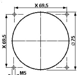
Bohrbild für Gerätestecker
