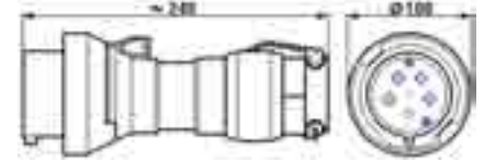
Stecker 5-polig
