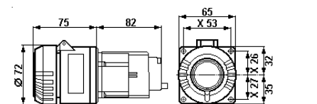
Prise à bride à 3 pôles
