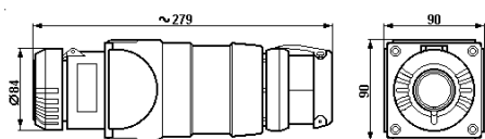
Prolongateur à 5 pôles
