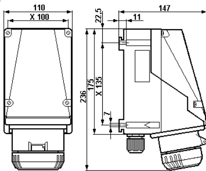
Prise murale à 4 pôles et 5 pôles
