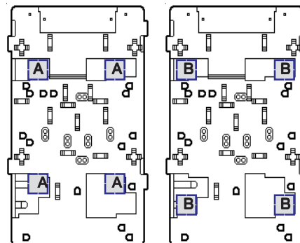
Befestigungspunkt A Steckdose 16A 3-pol.
