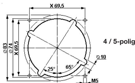
Bohrbild für Flanschsteckdose
