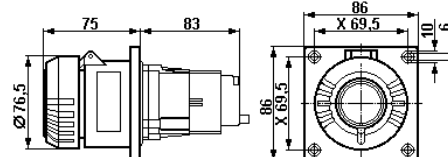
Flanschsteckdose 4-polig
