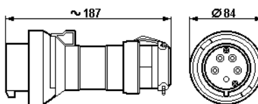
Stecker 5-polig
