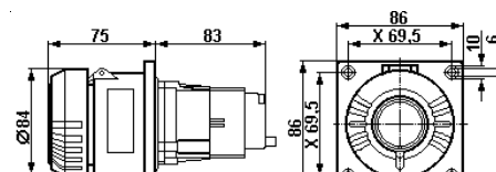
Flanschsteckdose 5-polig
