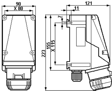
Wandsteckdose 3-polig
