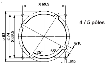
Gabarit de perçage pour prise à bride
