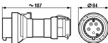
Fiche à 5 pôles
