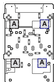
Point de fixation A Prise de 16A 3pôles
