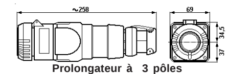
Prolongateur à 3 pôles
