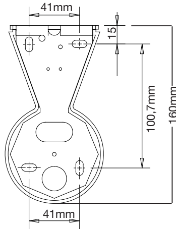
Abb. 1, Metallbügel des Wandauslegers / Metal bow of wall bracket
