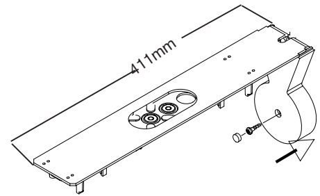
Abb. 2, Wandausleger / wall bracket
