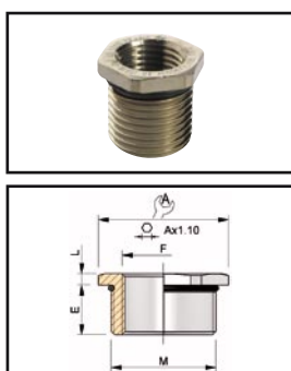
Réducteur laiton nickelé Male/Femelle Reducer nickel plated brass Male / Female
