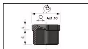
Bouchon / Plug
