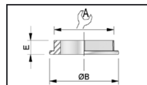
Contre-écrou Pg - ISO / Pg - ISO locknut
