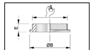
Contre-écrou Pg - ISO / Pg - ISO locknut
